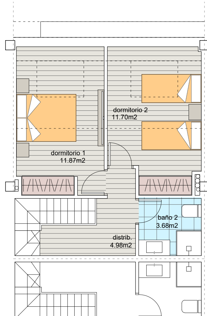
DÚPLEX ALTA
